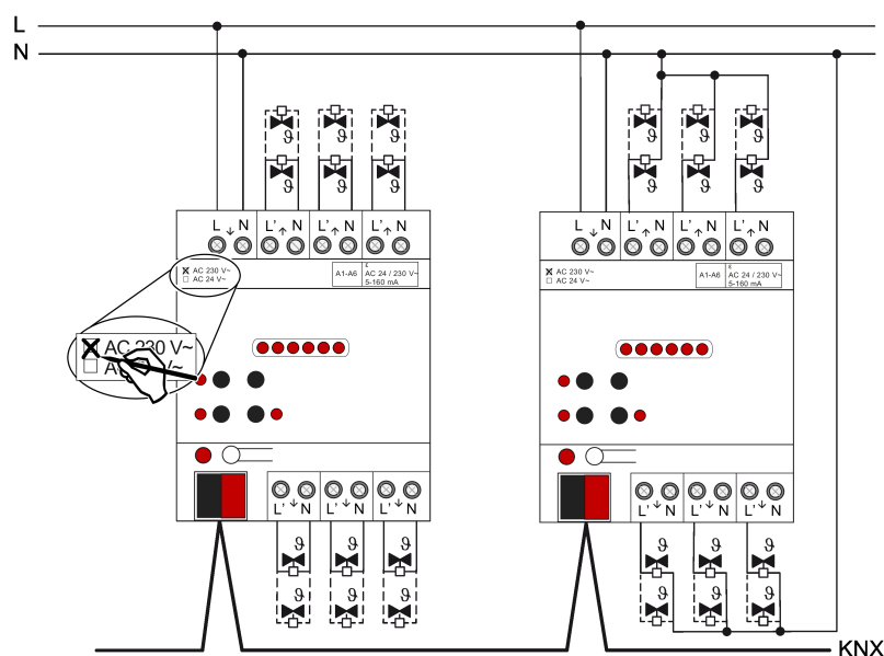
rysunek 3: Podłączenie siłowników AC 230 V (przykłady połączeń) po lewej: przewód neutralny siłowników poprowadzony oddzielnie do elementu wykonawczego / po prawej: wspólny przewód neutralny dla siłowników nastawczych
